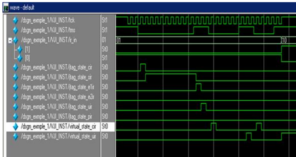
Figure 15. IR Shift Waveform
